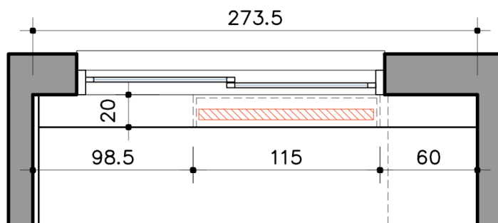
PAINEL - PLANTA
