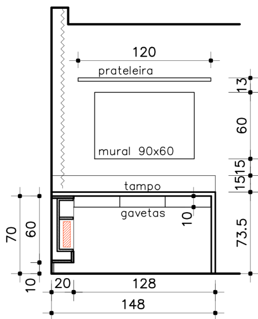
ESCRIVANINHA - VISTA
